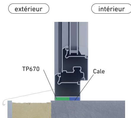
Figure 6 : Pose en partie basse sans rejingot
